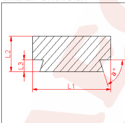
WIRBALIT® B Profil 14177
