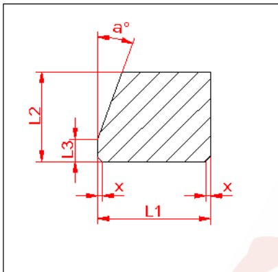
WIRBALIT® B Profil 13946
